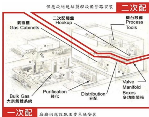
圖二、廠房氣體供應系統
